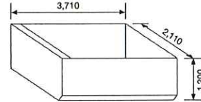
8m³コンテナ
